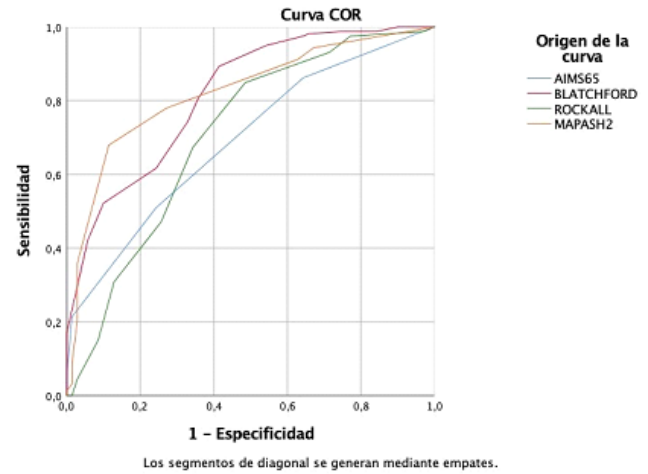
FIGURA 1 Curva ROC.
