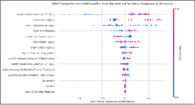
Figura 1. Gráfico SHAP Beeswarm del modelo de predicción de respuesta clínica a la semana 26.
